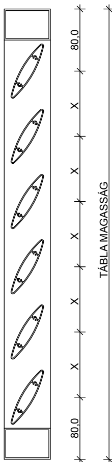
Ellipsun80 lamella és 60x40 alumínium keret
