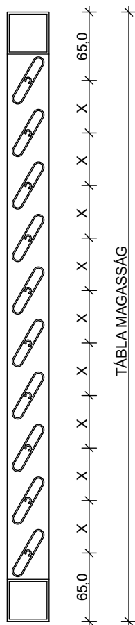
Ellipsun50 lamella és 40x40 alumínium keret
